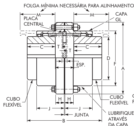
Tipo GL20 – 1 Capa de dentes padrão para placa central de cubos padrão invertidos
