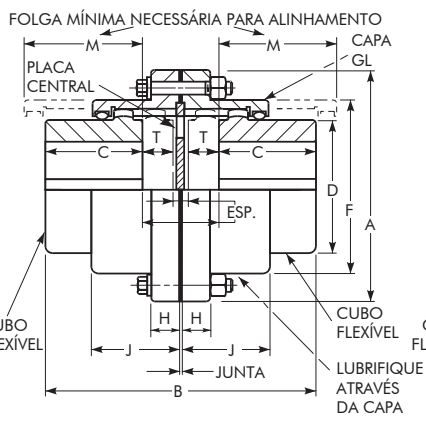
Tipo GL20 – 2 Capa de dentes longa para placa central de cubos longos de corte
