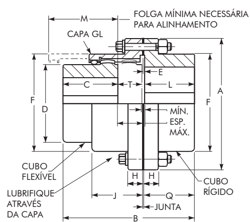
Tipo GL52-2 Capa de dentes longa para placa central de cubos longos de corte
