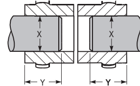
Engrenamento simples
