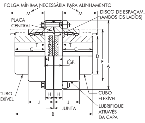
Tipo GL20 – 4 Capa de dentes padrão para placa central de cubos padrão invertidos
