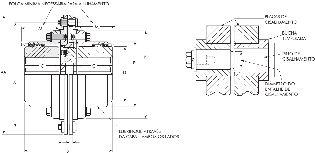
Dimensões (mm)
