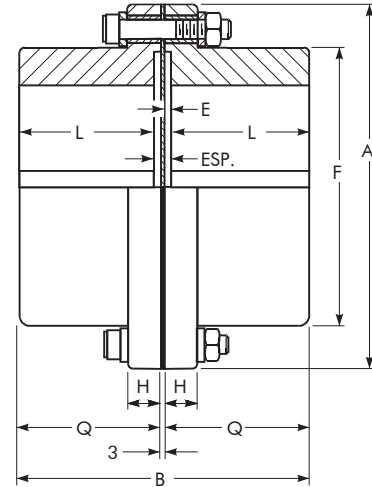
Acoplamento rígido Tipo GP82
