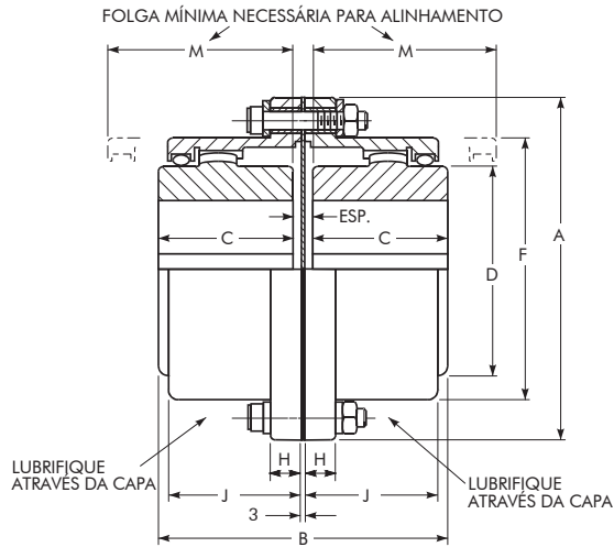
Dimensões (mm)
