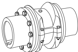
Tipo T31 com espaçador inteiro
