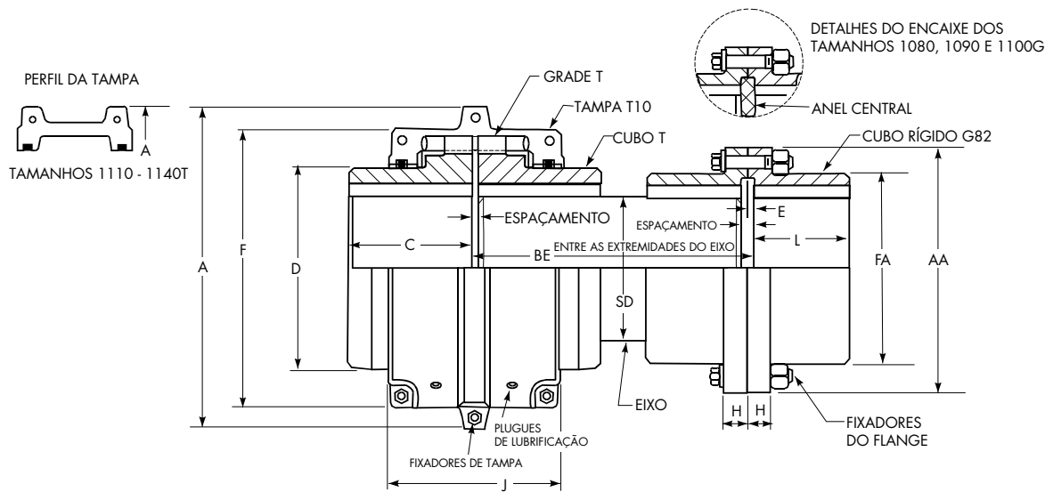
Dimensões (mm)
