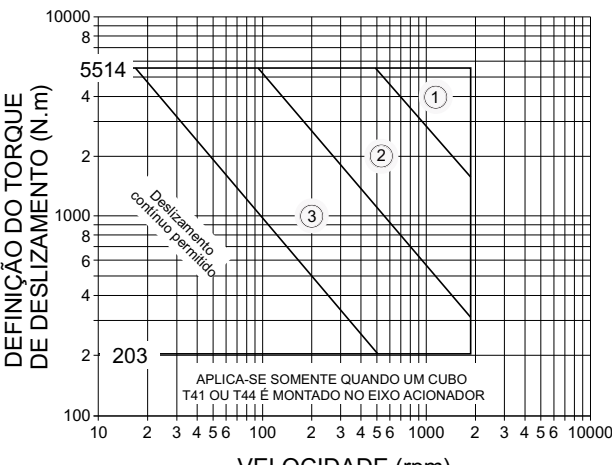
TAMANHOS 1110T41 E 1110T44
