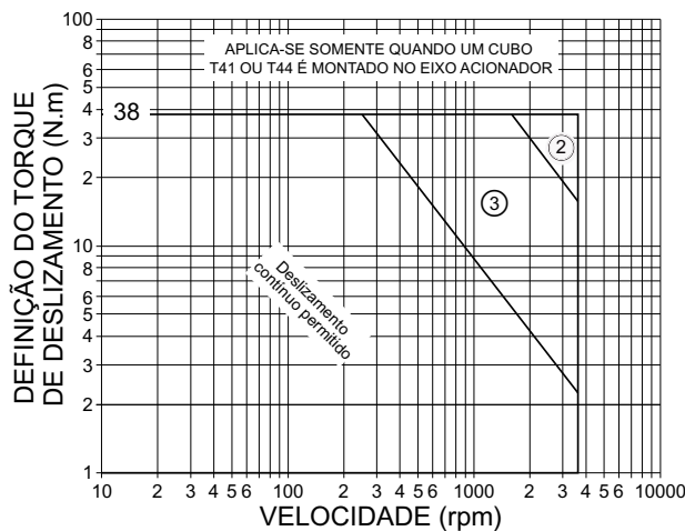
TAMANHOS 1020T41 E 1020T44
